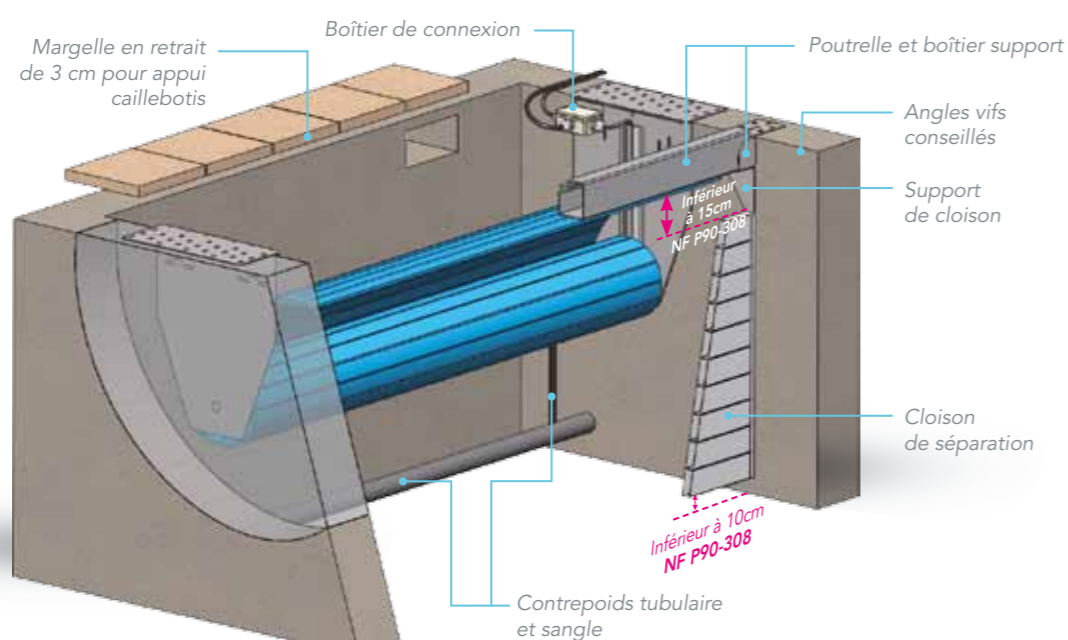
Exemple avec cloison de séparation en PVC et flasques montées sur supports plats fixés sur l'arase
